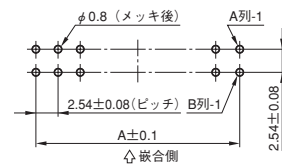
基板取付穴寸法(参考・装着面)
