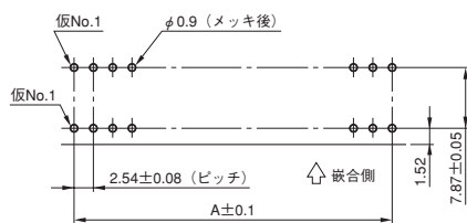
基板取付穴寸法(参考)
